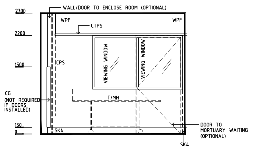
ELEVATION 4
