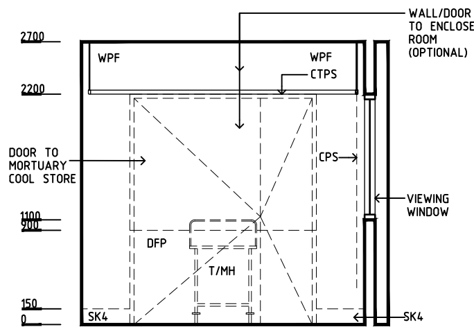
ELEVATION 3
