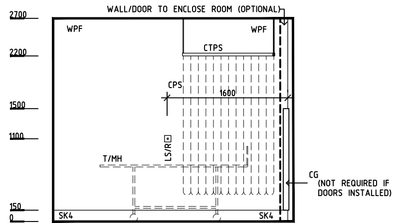
ELEVATION 2
