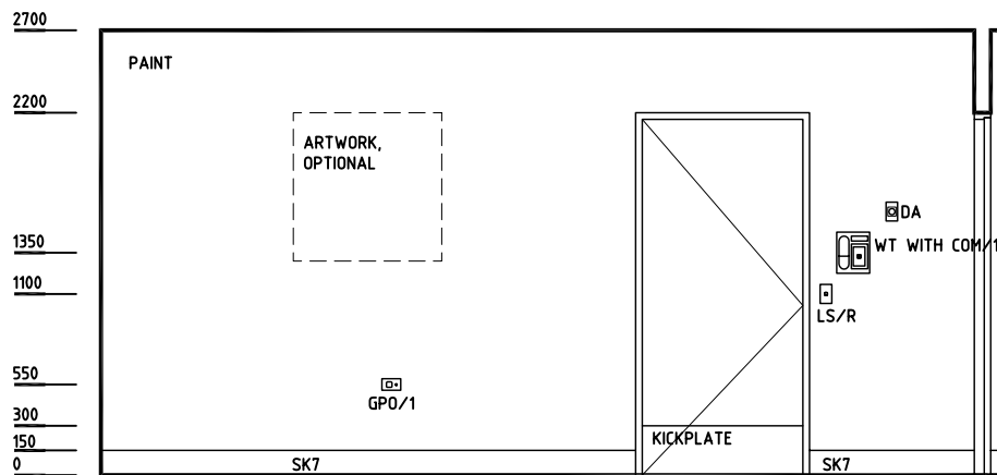
ELEVATION 1
