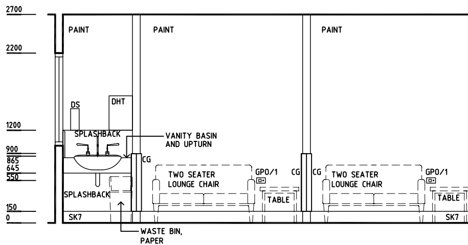
ELEVATION 3
