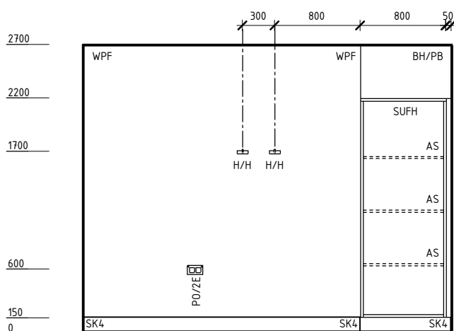
ELEVATION 3
