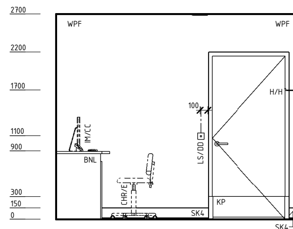
ELEVATION 2
