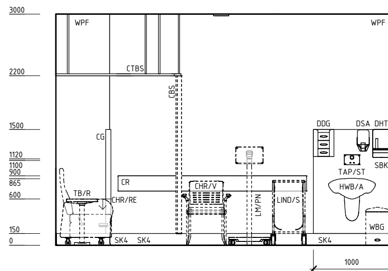
ELEVATION 2
