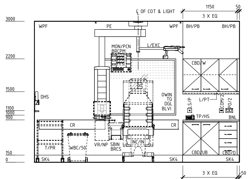
ELEVATION 4
