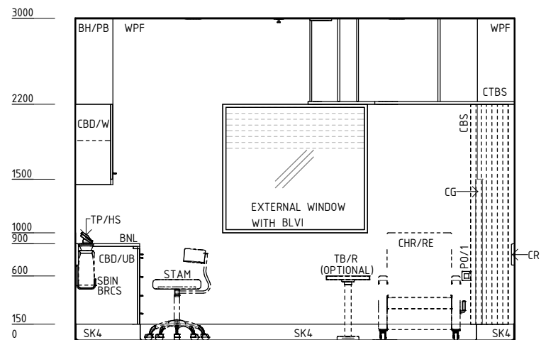
ELEVATION 1
