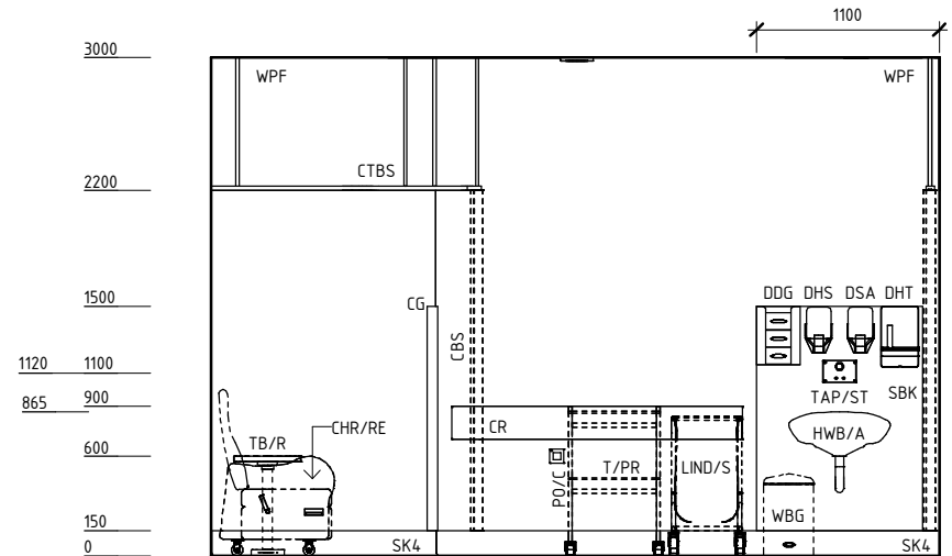
ELEVATION 2
