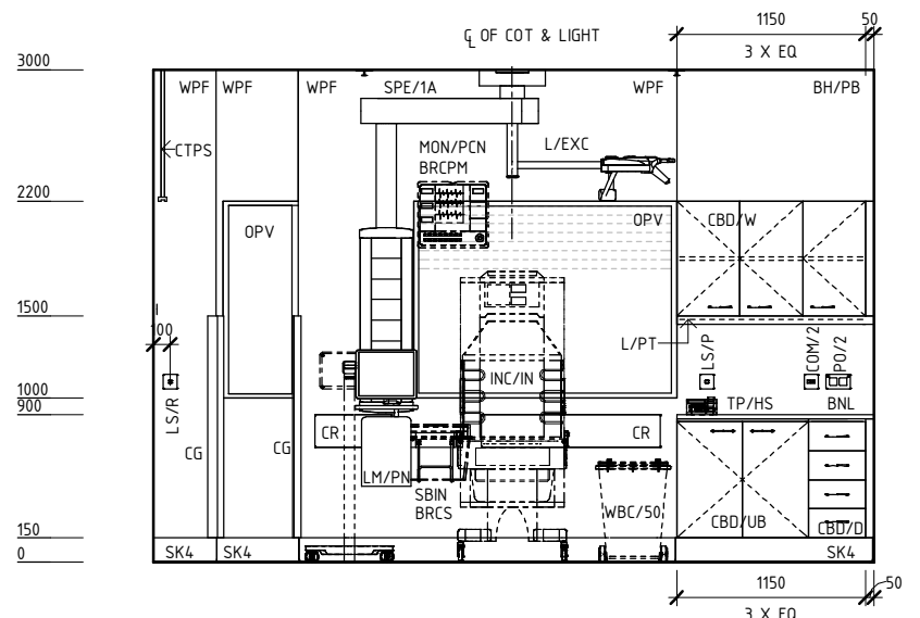
ELEVATION 4
