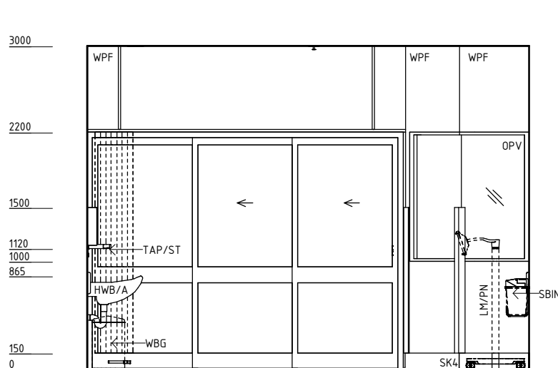
ELEVATION 3
