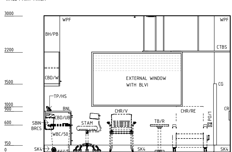
ELEVATION 1
