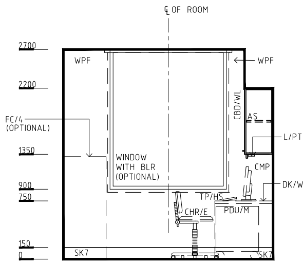
ELEVATION 1
