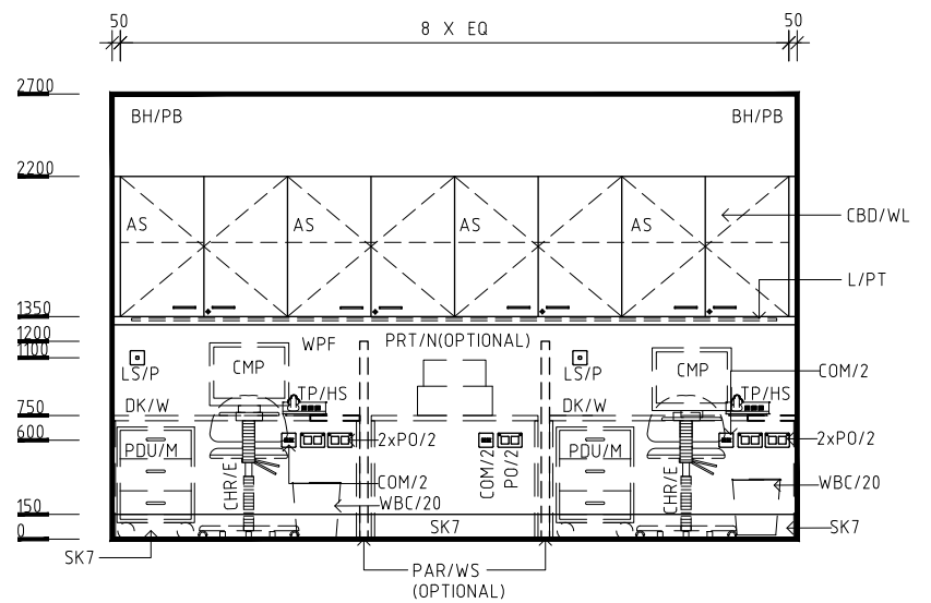
ELEVATION 2
