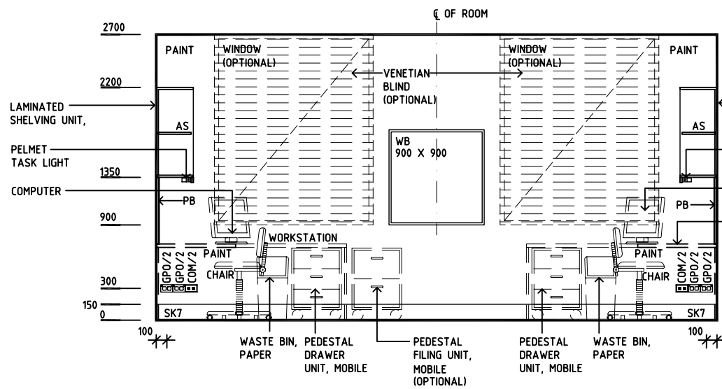
ELEVATION 1
