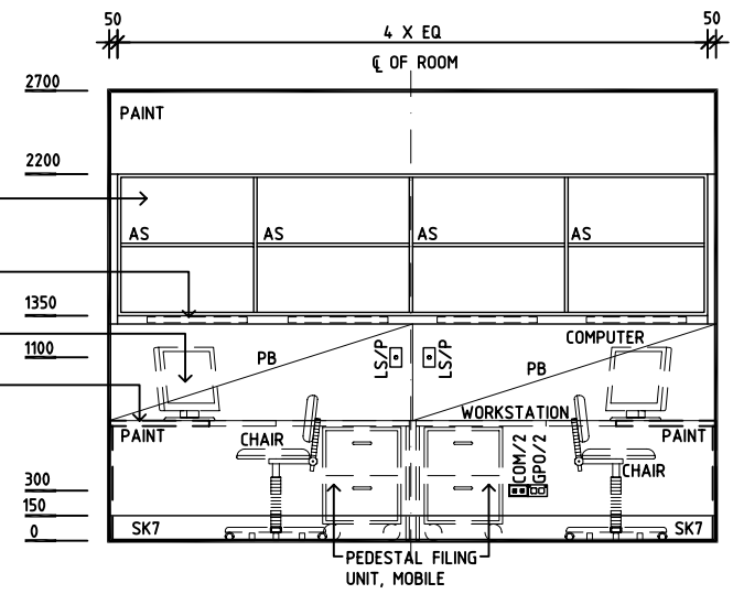
ELEVATION 2
