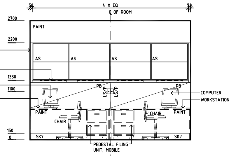
ELEVATION 4
