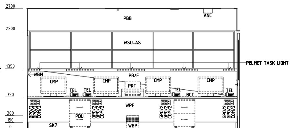
ELEVATION 2
