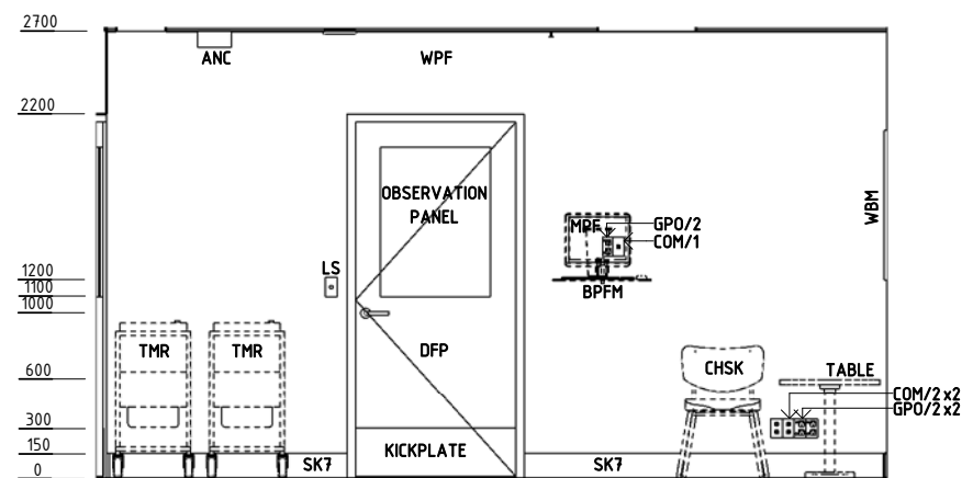
ELEVATION 4
