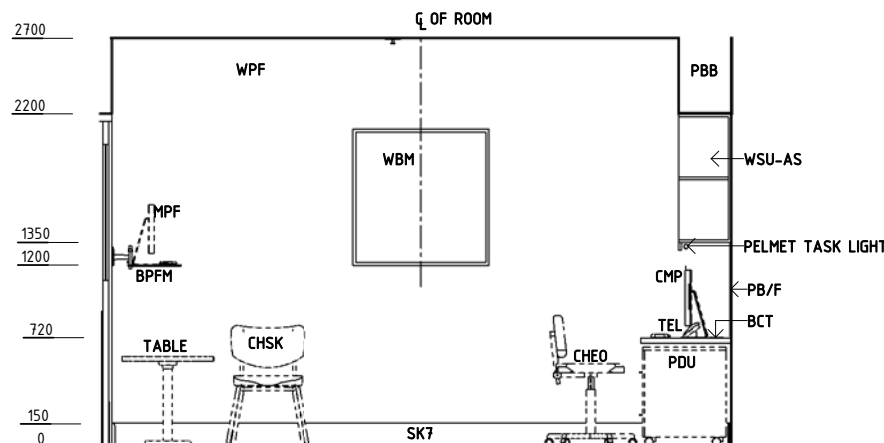
ELEVATION 1
