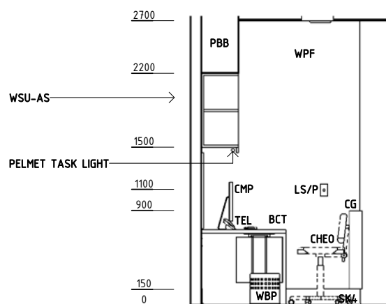
ELEVATION 3
