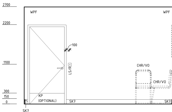
ELEVATION 3
