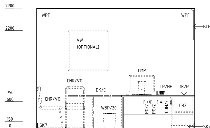
ELEVATION 4
