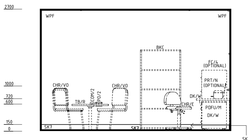
ELEVATION 4
