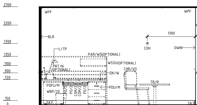
ELEVATION 2
