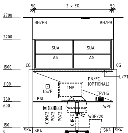
ELEVATION 2
