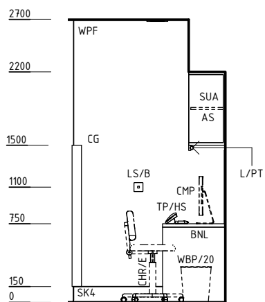
ELEVATION 1
