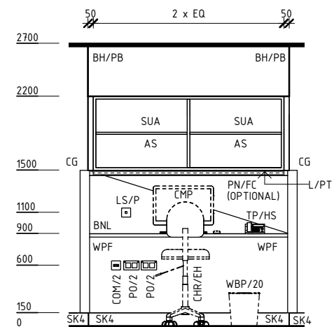
ELEVATION 2
