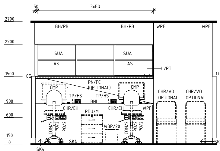
ELEVATION 2
