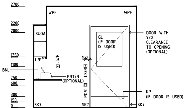
ELEVATION 3
