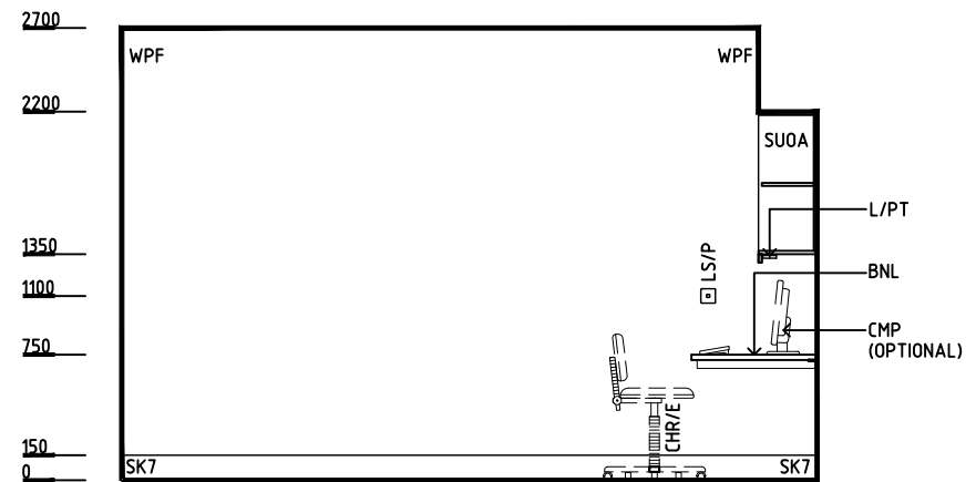
ELEVATION 4
