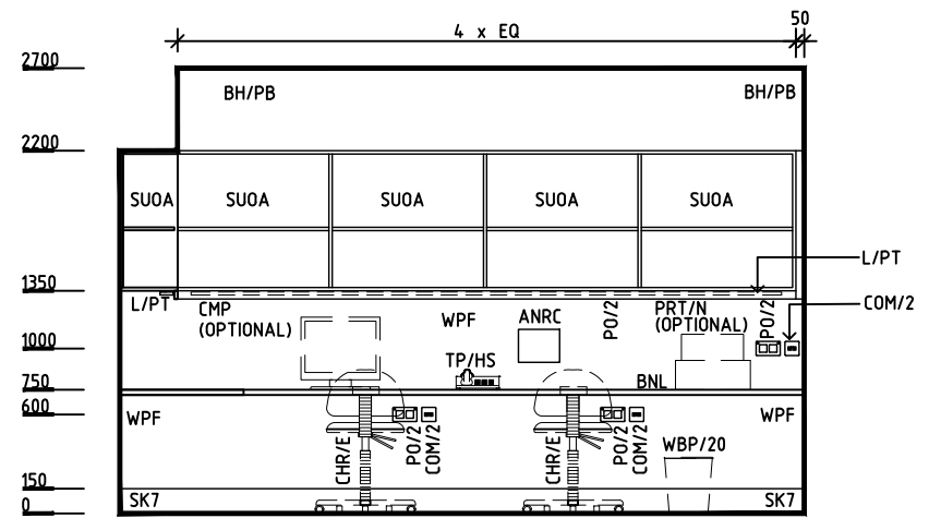
ELEVATION 2
