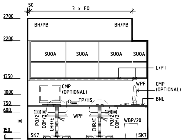
ELEVATION 1
