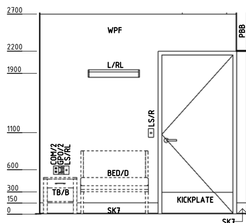
ELEVATION 3
