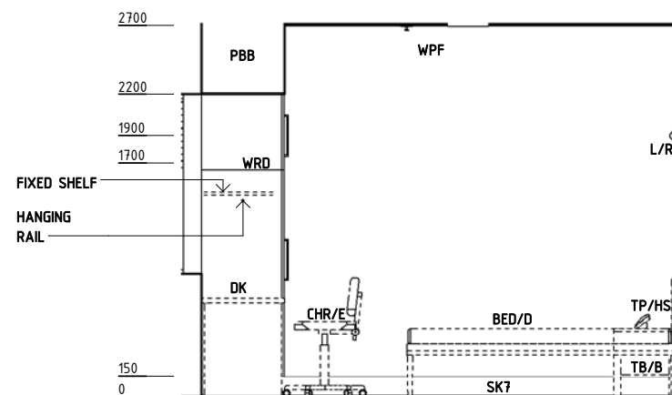
ELEVATION 2
