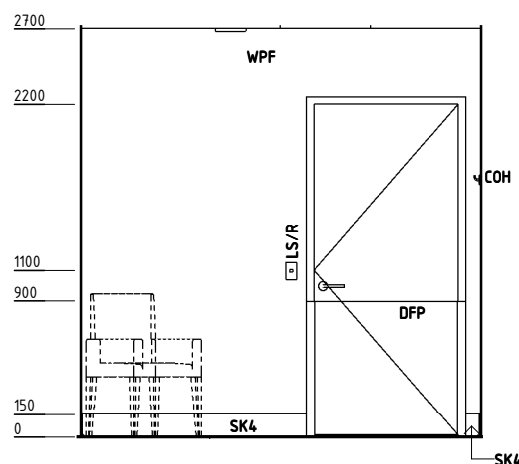
ELEVATION 3
