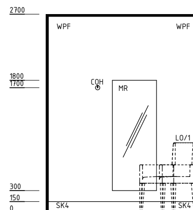
ELEVATION 4
