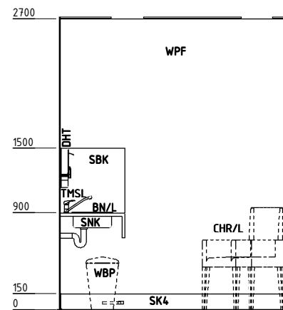
ELEVATION 2
