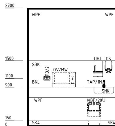
ELEVATION 2
