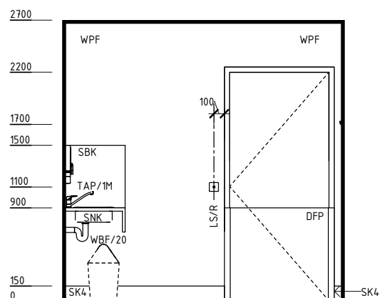
ELEVATION 3
