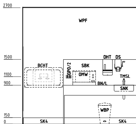
ELEVATION 1
