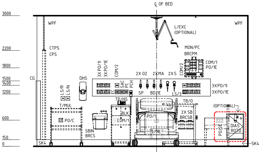
ELEVATION 4
