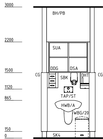
ELEVATION 5
