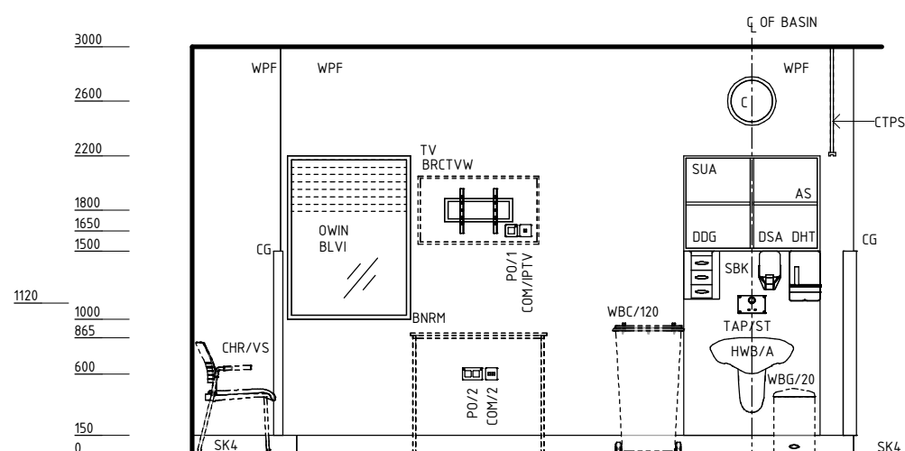
ELEVATION 2
