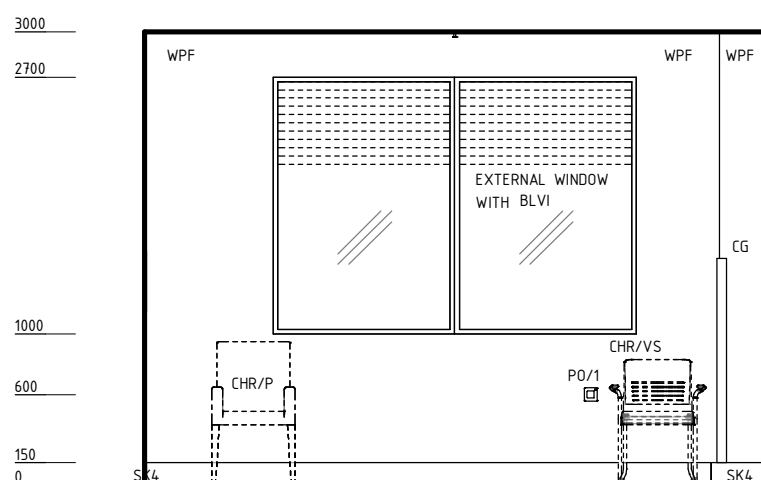
ELEVATION 1
