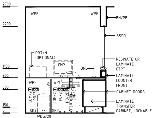
ELEVATION 4
