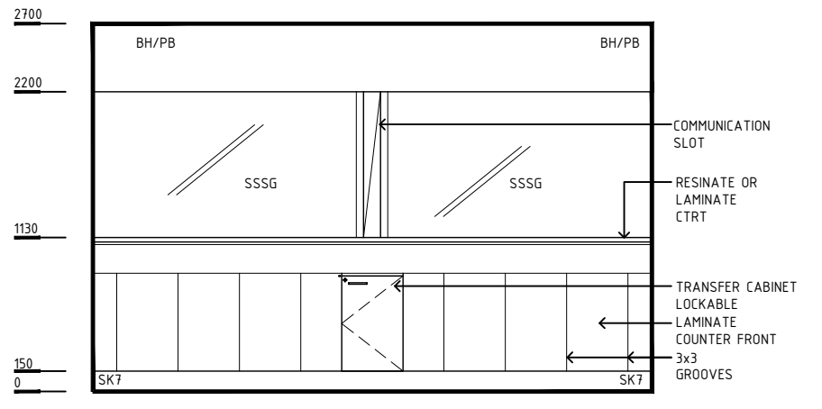
ELEVATION 5
