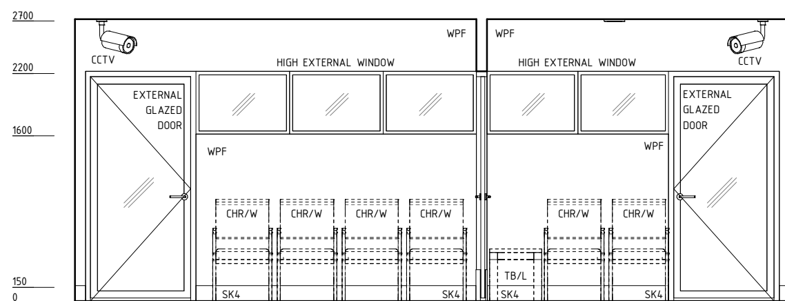
ELEVATION 3
