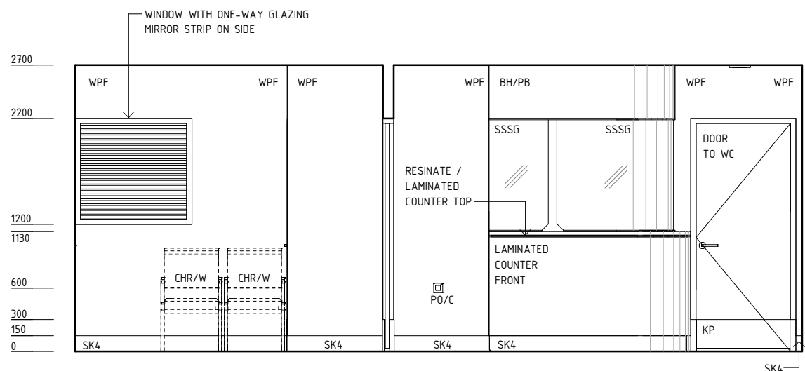
ELEVATION 1
