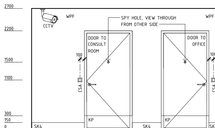
ELEVATION 5
