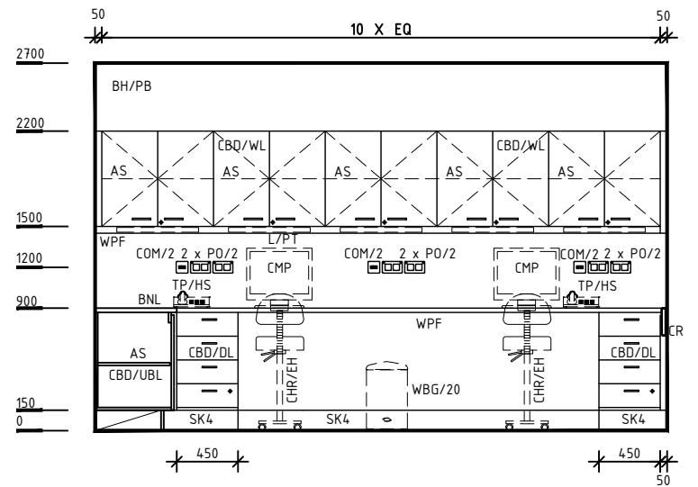
ELEVATION 2
