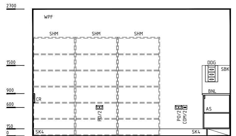
ELEVATION 4
