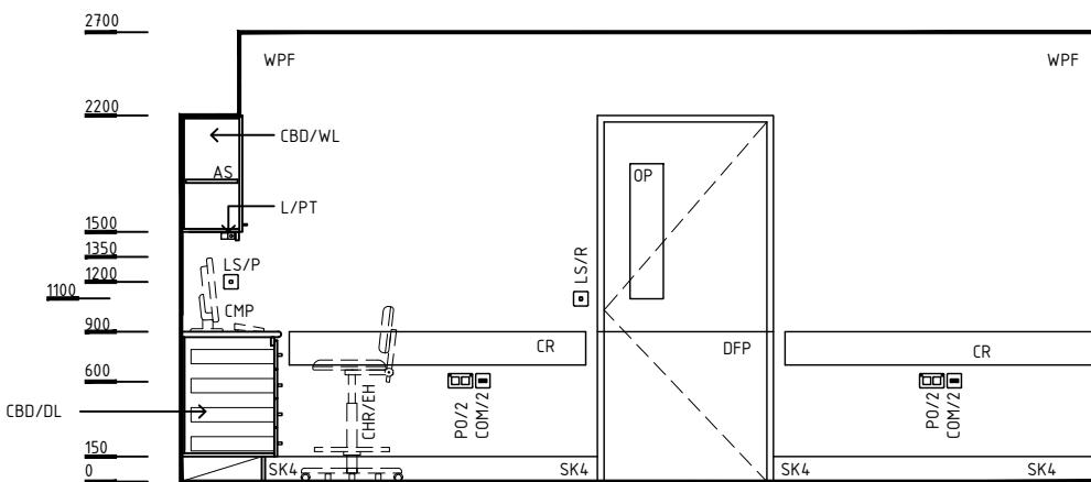
ELEVATION 3
