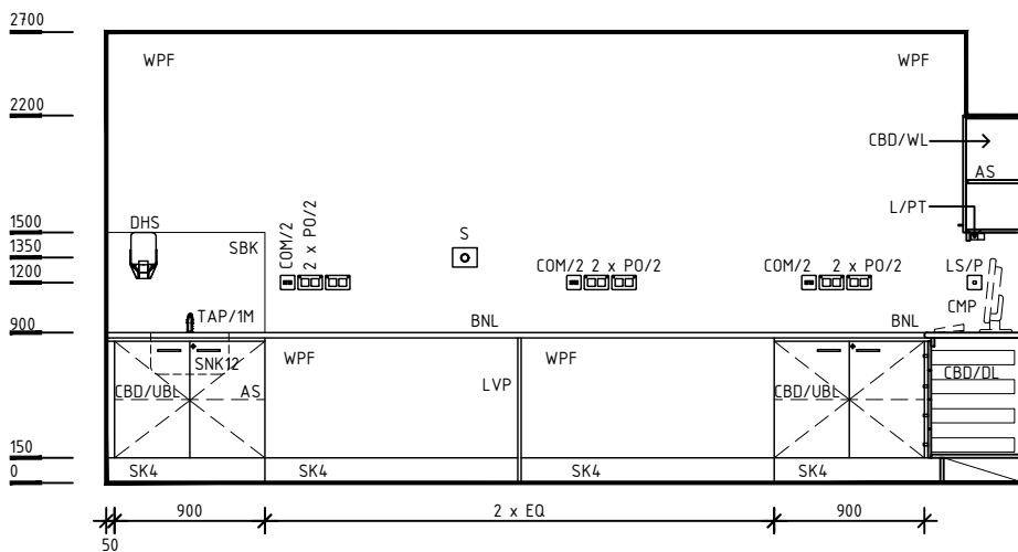
ELEVATION 1
