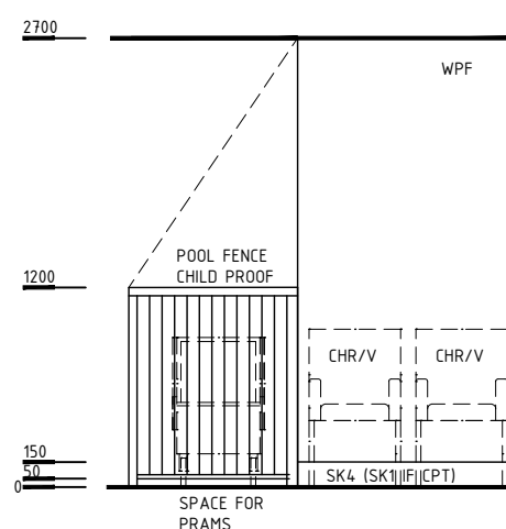
ELEVATION 4
