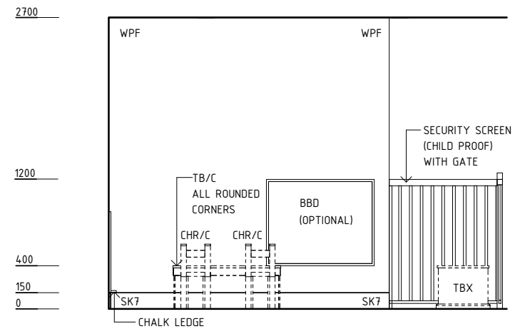
ELEVATION 2
