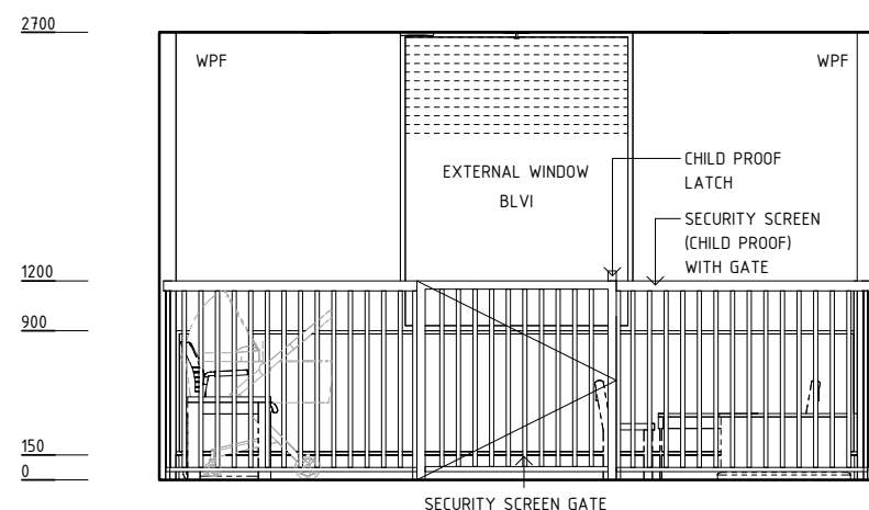
ELEVATION 3
