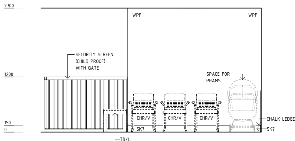
ELEVATION 4
