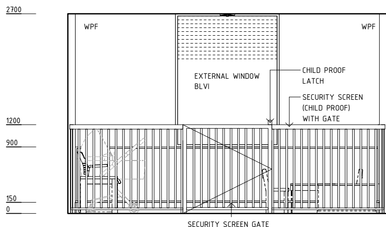
ELEVATION 3
