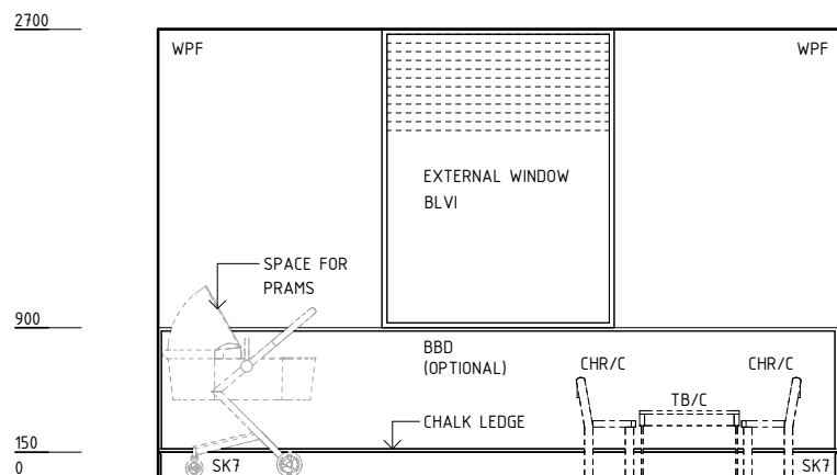
ELEVATION 1
