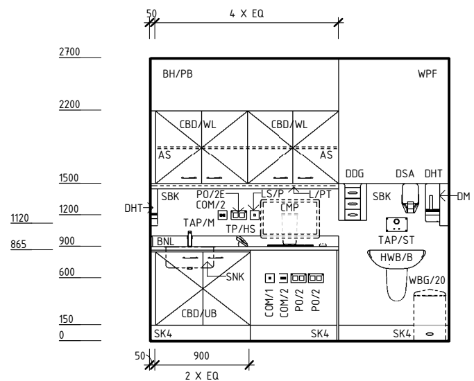
ELEVATION 2
