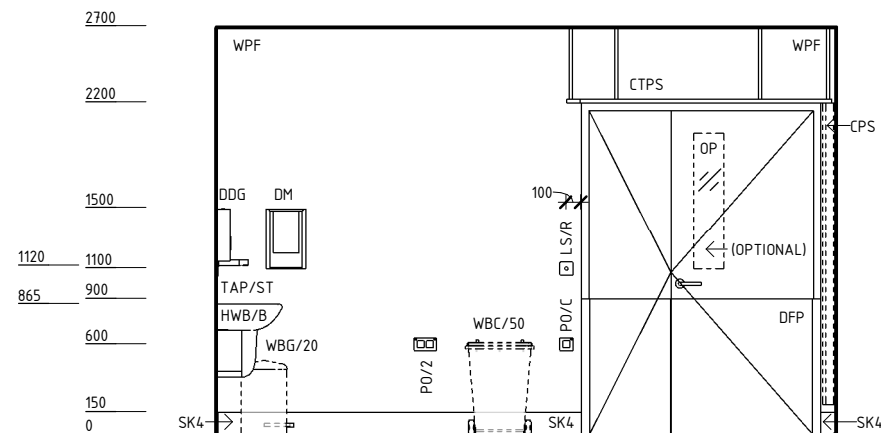
ELEVATION 3
