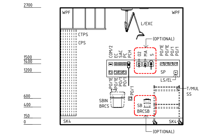
ELEVATION 4
