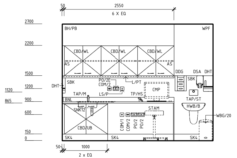
ELEVATION 2
