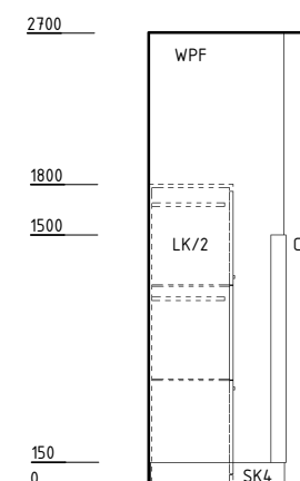
ELEVATION 3
