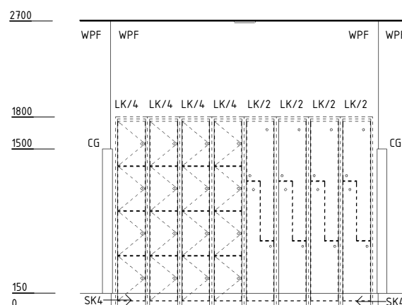
ELEVATION 2
