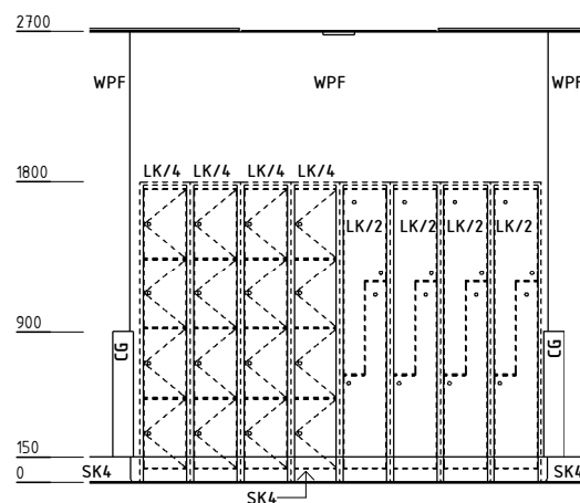
ELEVATION 2
