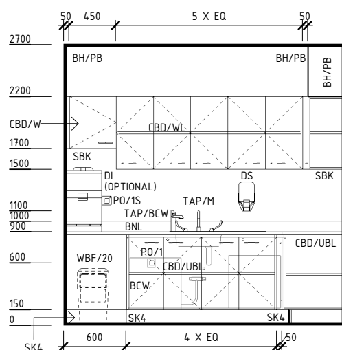
ELEVATION 1
