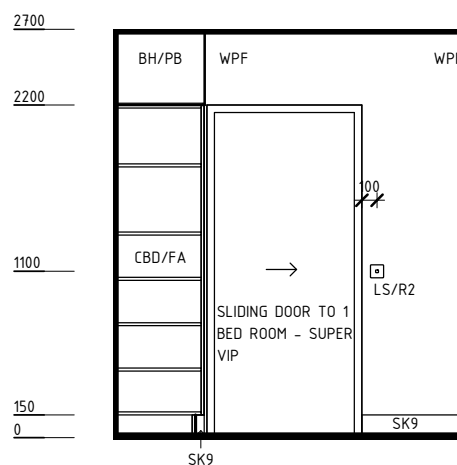
ELEVATION 2
