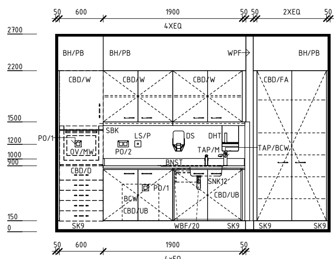
ELEVATION 1
