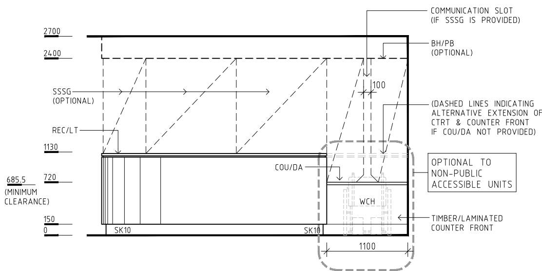
ELEVATION 1
