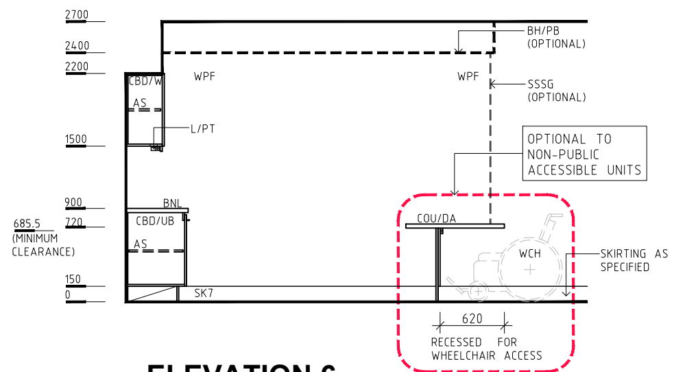
ELEVATION 6
