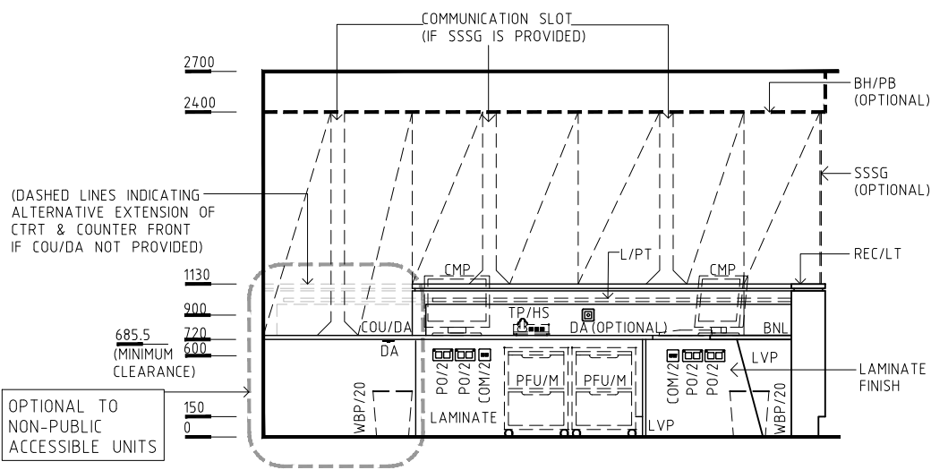
ELEVATION 3
