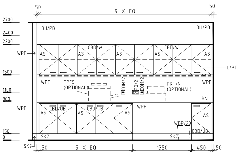
ELEVATION 5
