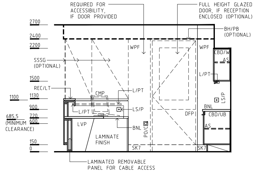
ELEVATION 4
