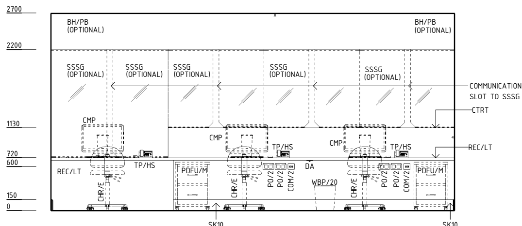
ELEVATION 3
