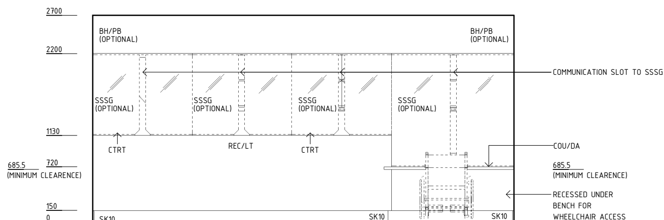
ELEVATION 5
