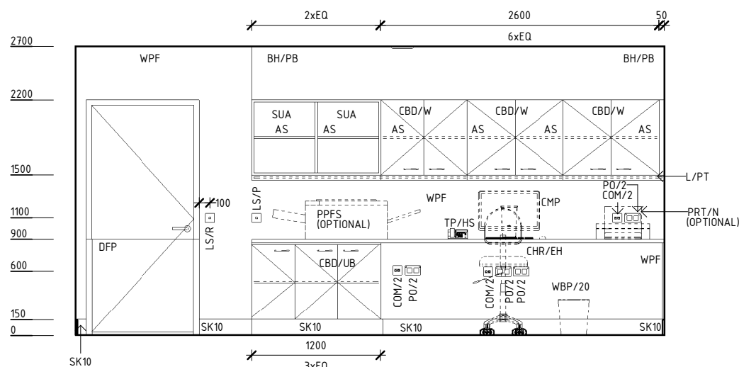
ELEVATION 1
