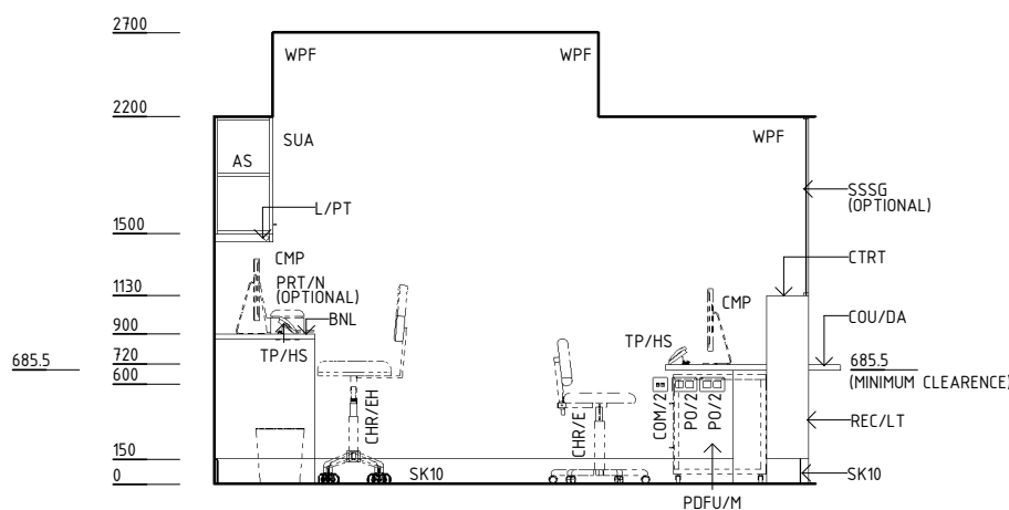
ELEVATION 2
