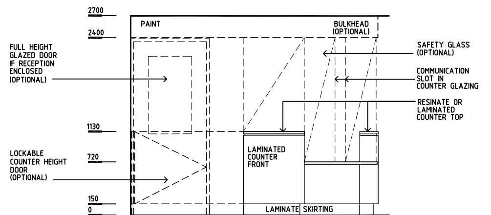
ELEVATION 2
