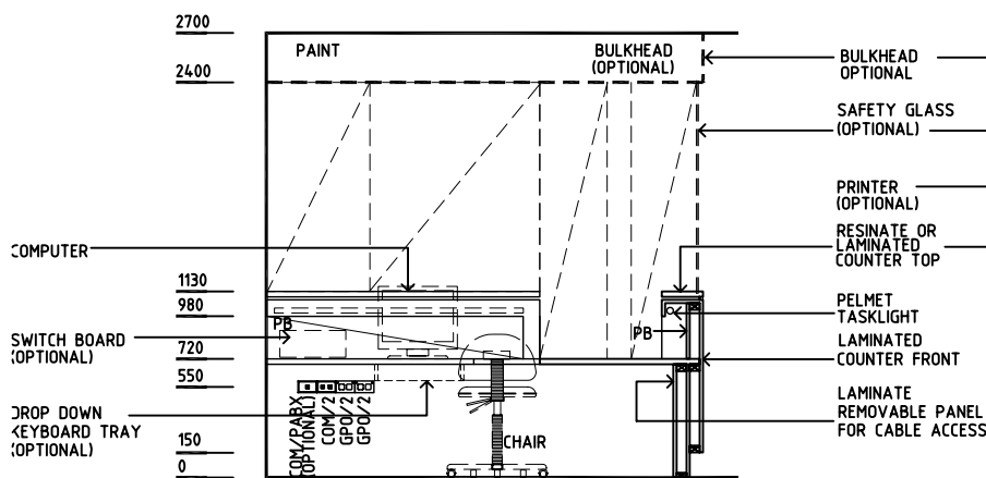
ELEVATION 3
