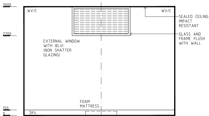
ELEVATION 1
