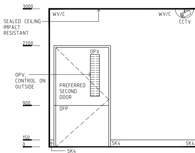
ELEVATION 2
