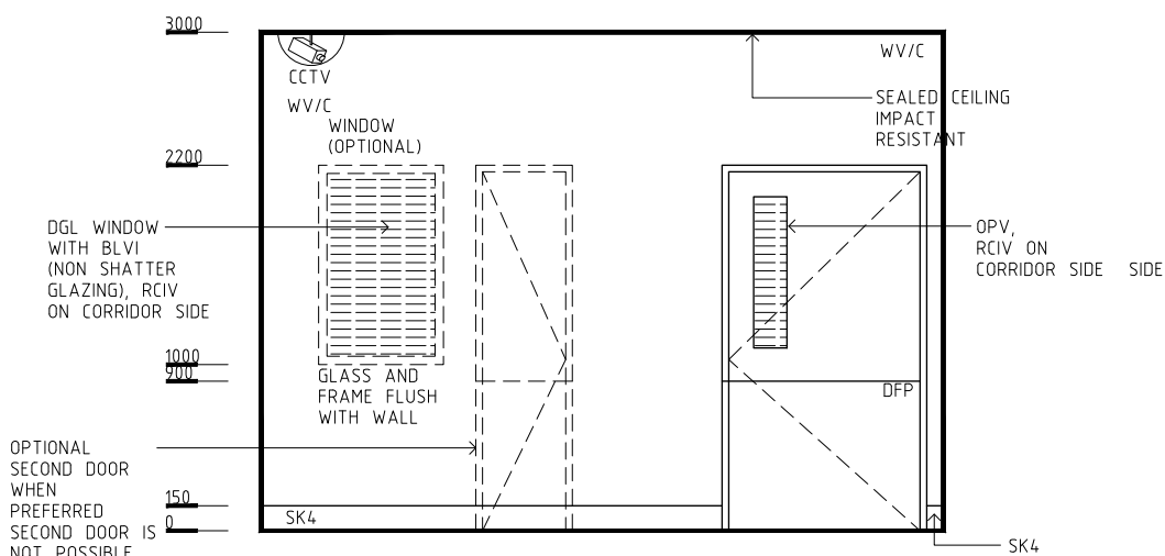
ELEVATION 3
