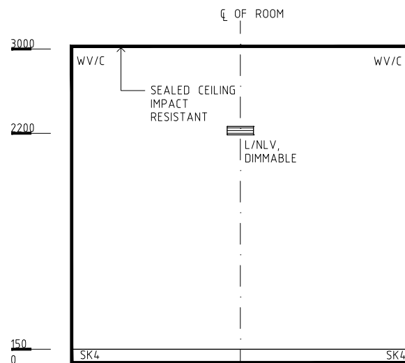
ELEVATION 4
