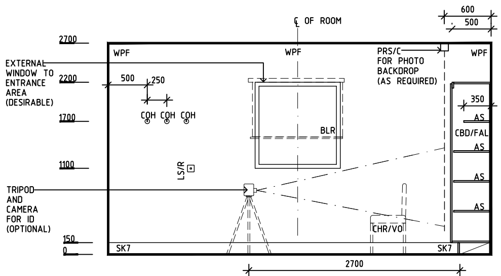
ELEVATION 4
