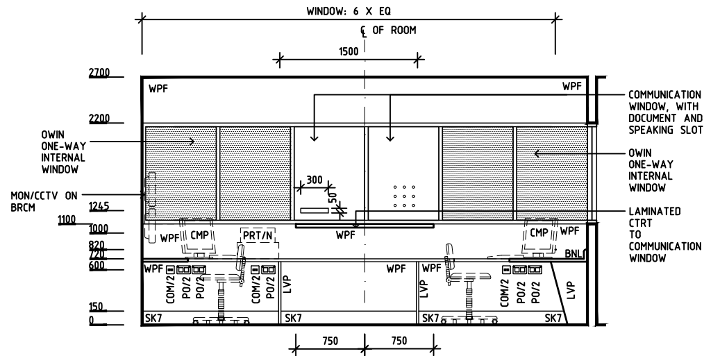
ELEVATION 2
