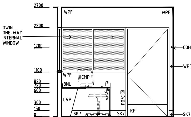
ELEVATION 3
