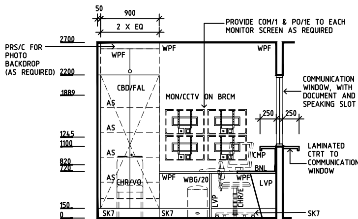
ELEVATION 1
