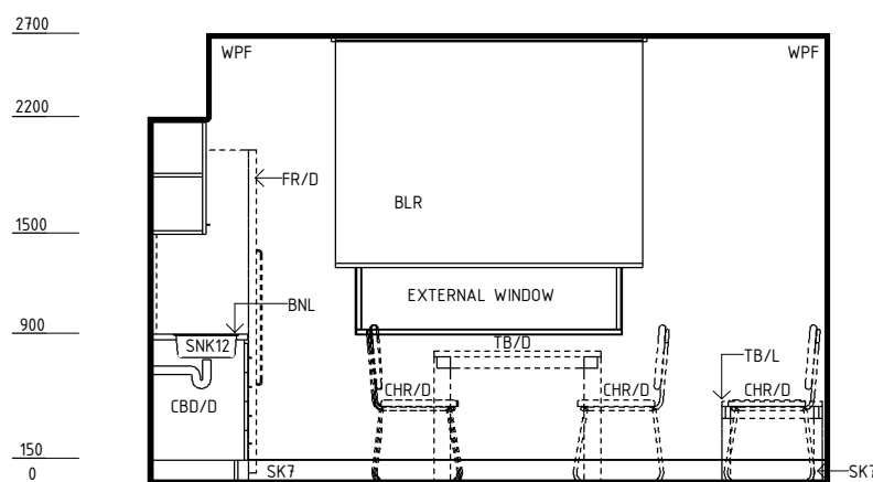
ELEVATION 1
