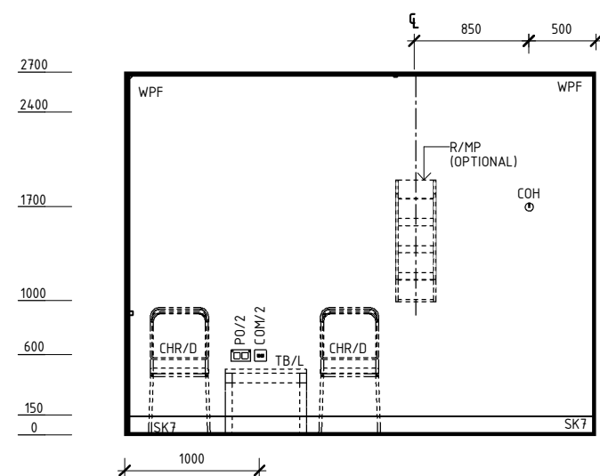
ELEVATION 2
