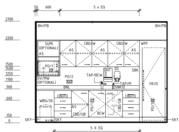
ELEVATION 4
