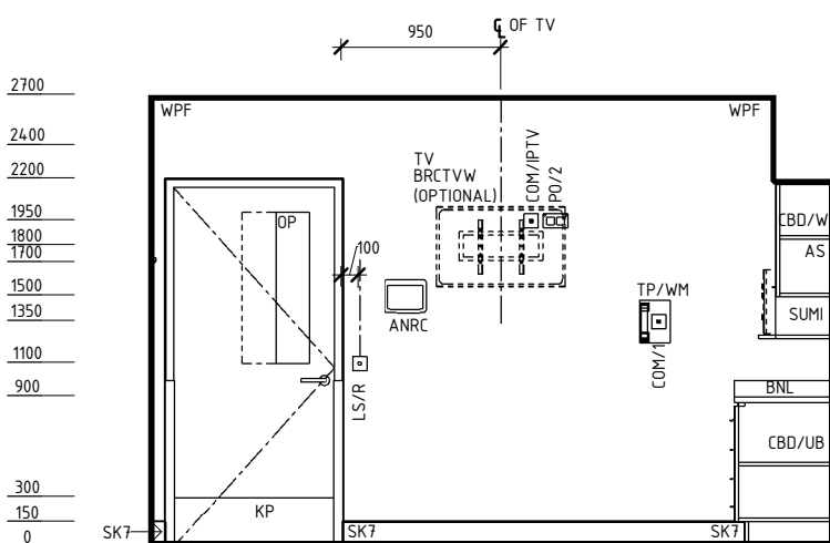
ELEVATION 3
