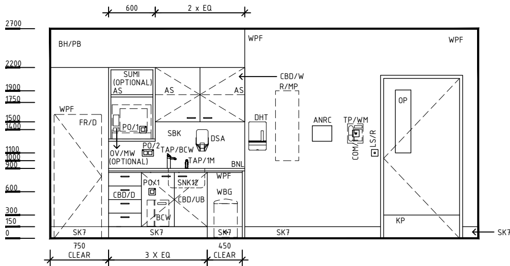
ELEVATION 3
