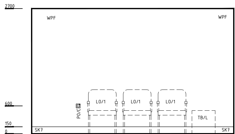
ELEVATION 4
