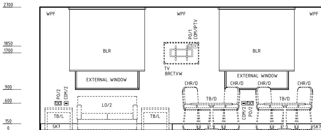
ELEVATION 1
