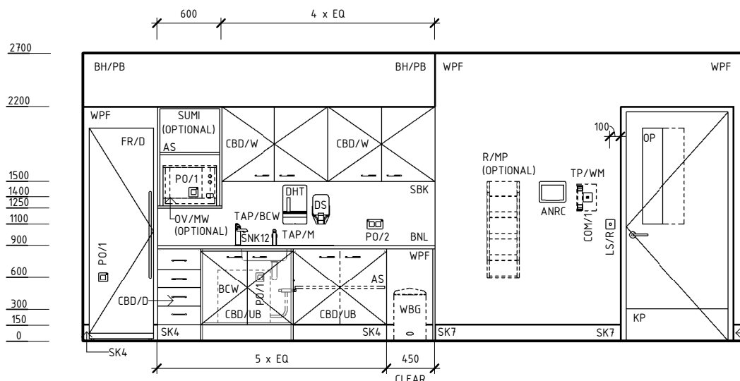
ELEVATION 3
