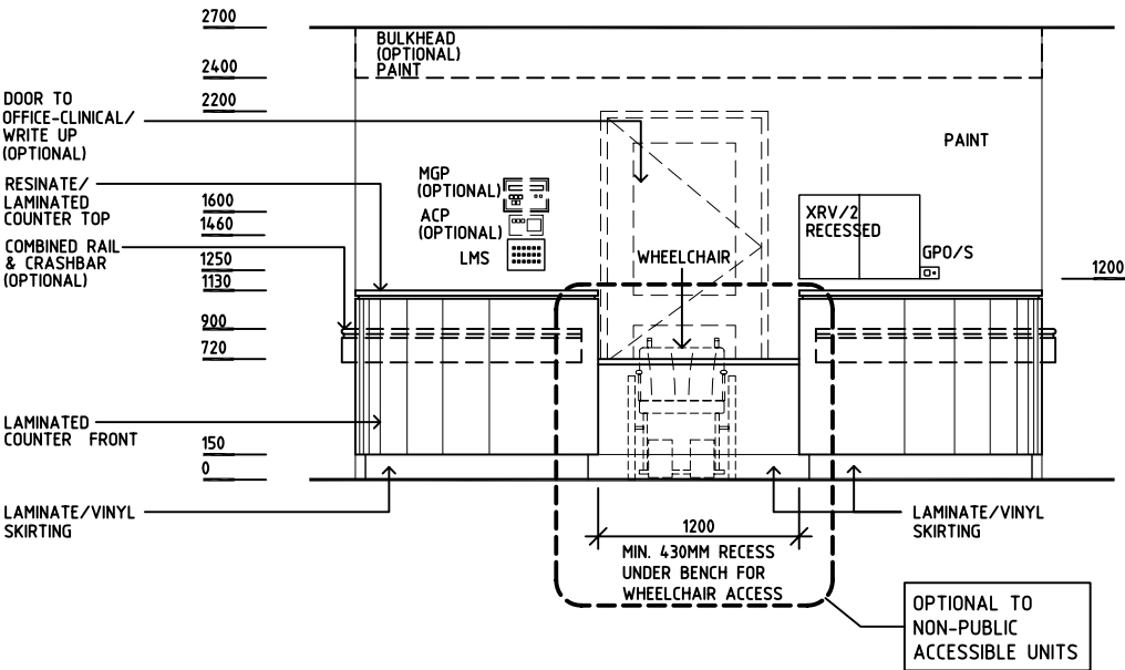
ELEVATION 2
