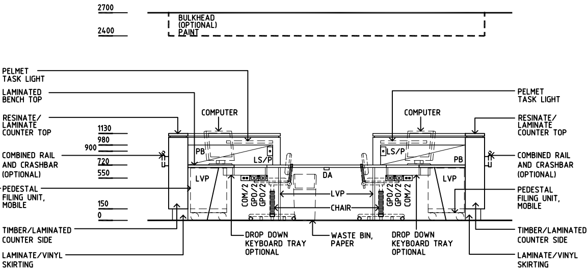
ELEVATION 5
