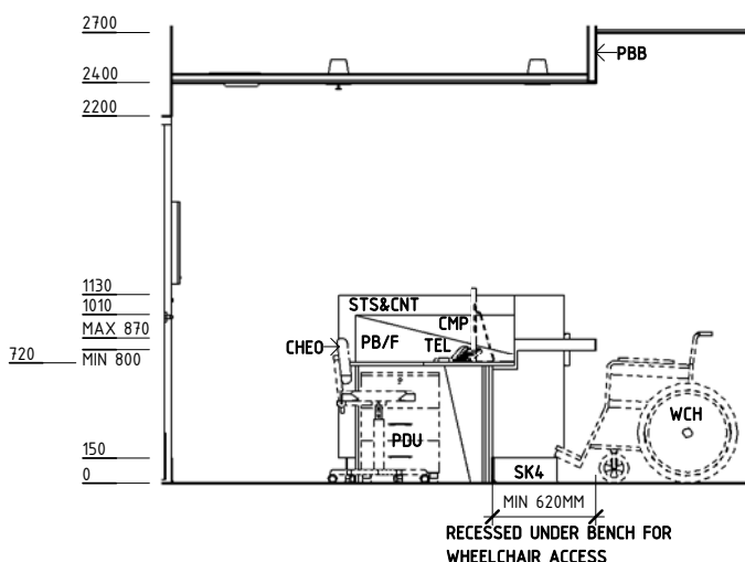
ELEVATION 4
