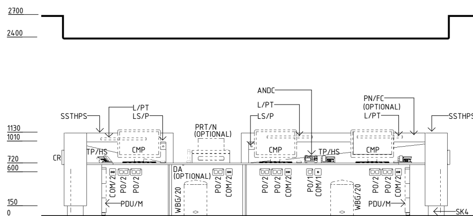
ELEVATION 5
