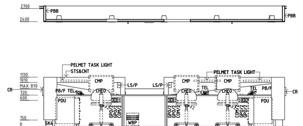
ELEVATION 3
