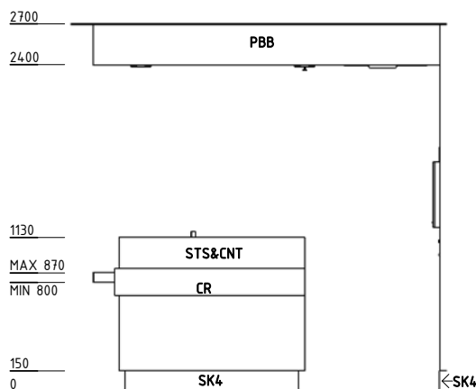
ELEVATION 1
