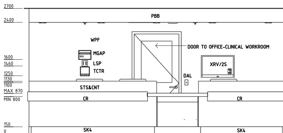
ELEVATION 2
