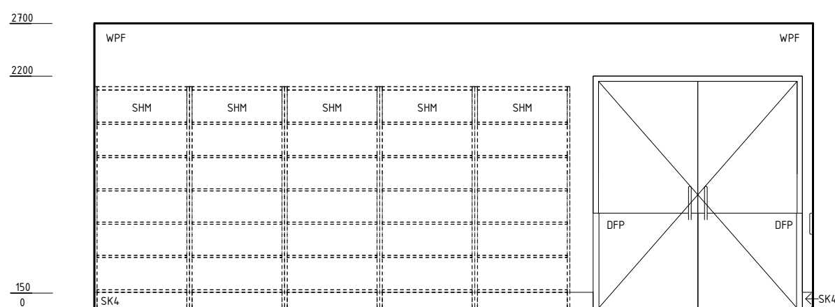
ELEVATION 1
