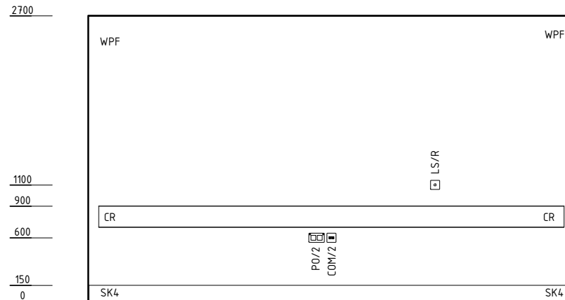
ELEVATION 2
