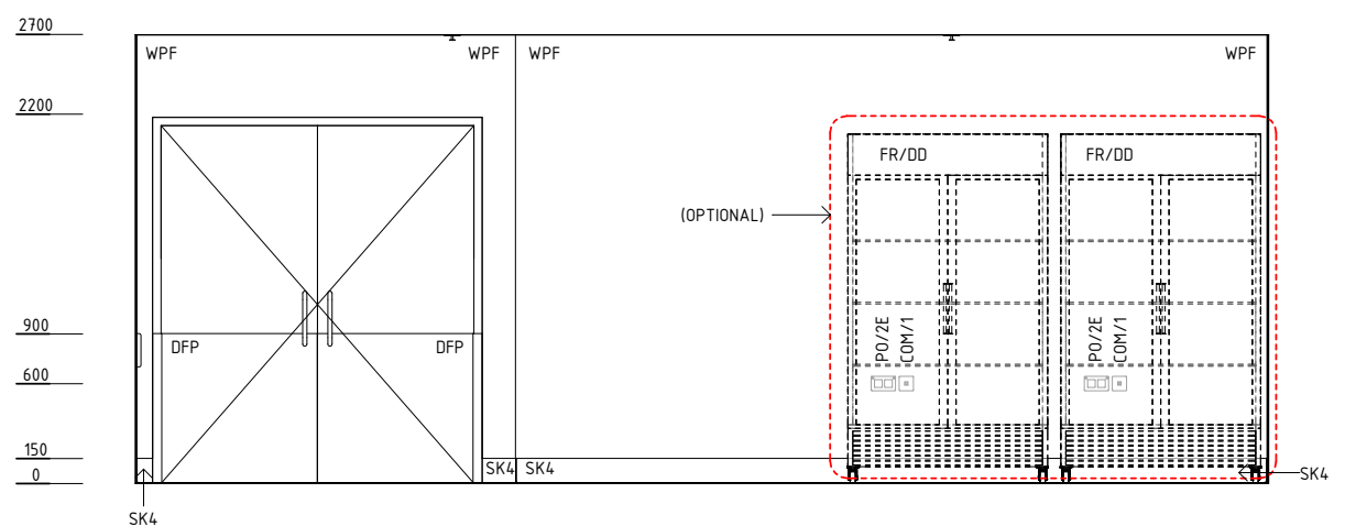
ELEVATION 3
