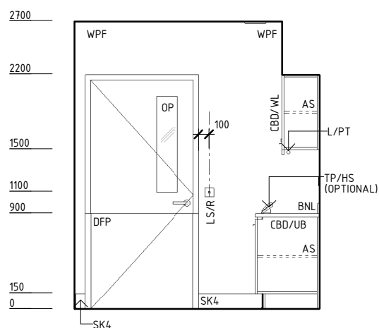
ELEVATION 3
