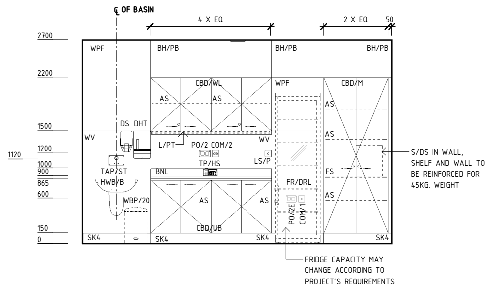
ELEVATION 4
