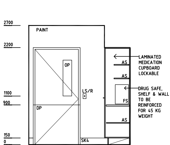
ELEVATION 3
