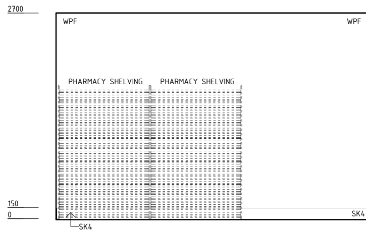
ELEVATION 2
