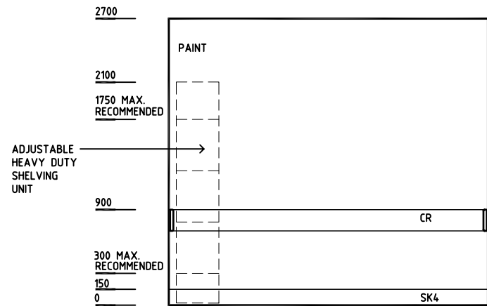
ELEVATION 1
