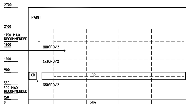
ELEVATION 4
