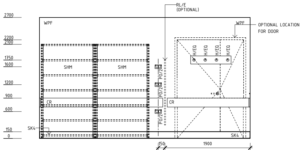
ELEVATION 2
