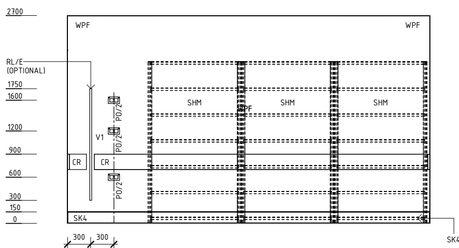
ELEVATION 4
