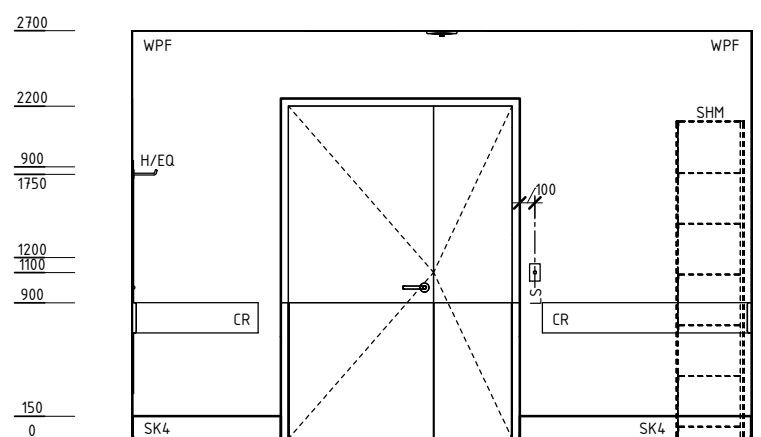
ELEVATION 3
