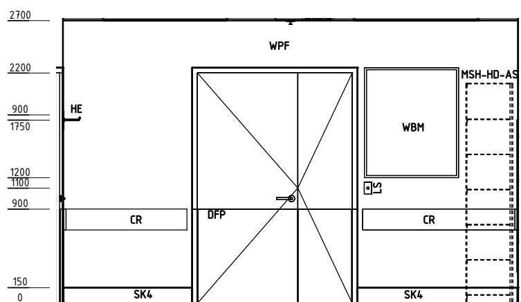
ELEVATION 3
