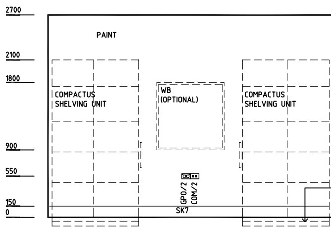
ELEVATION 1
