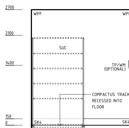
ELEVATION 5
