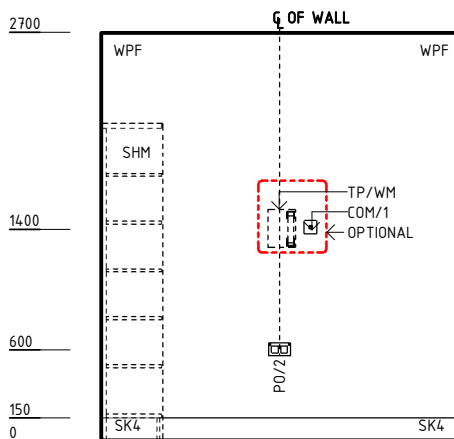
ELEVATION 2
