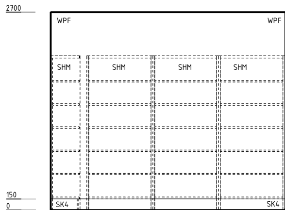
ELEVATION 1
