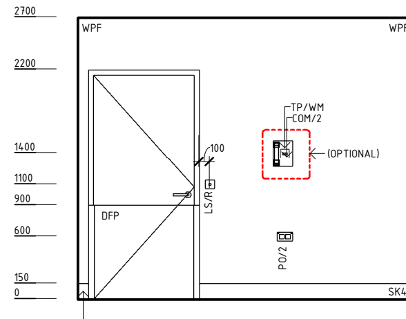
ELEVATION 6
