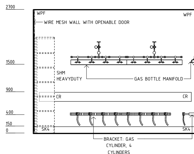
ELEVATION 4
