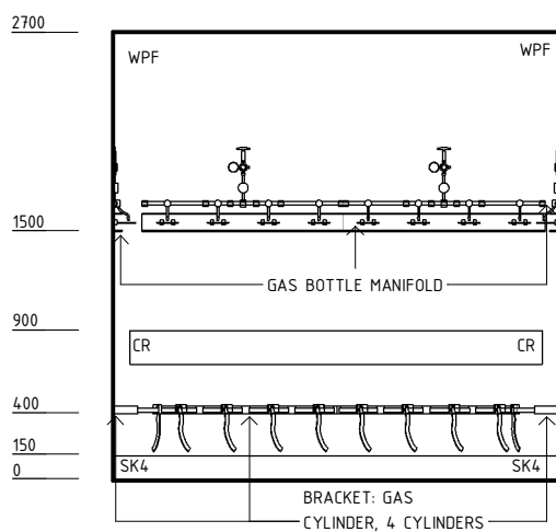
ELEVATION 1
