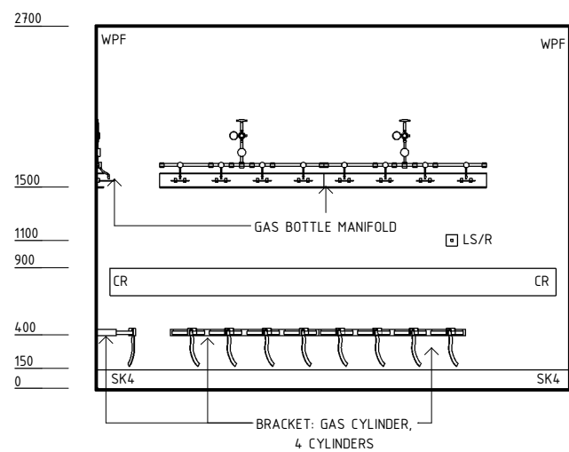
ELEVATION 2
