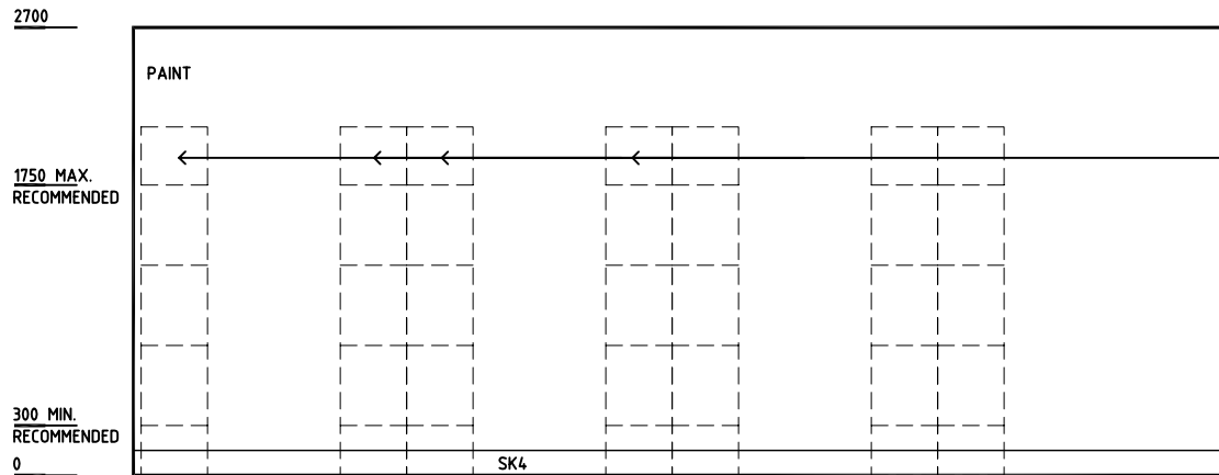
ELEVATION 1
