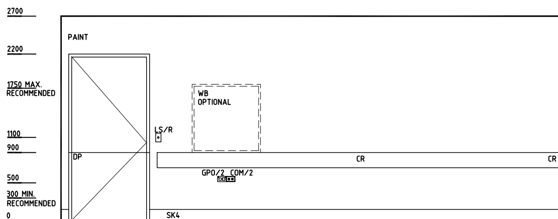
ELEVATION 3
