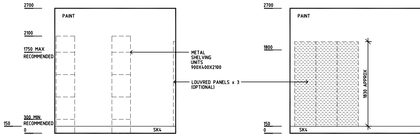
ELEVATION 1
