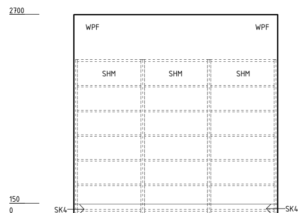
ELEVATION 4
