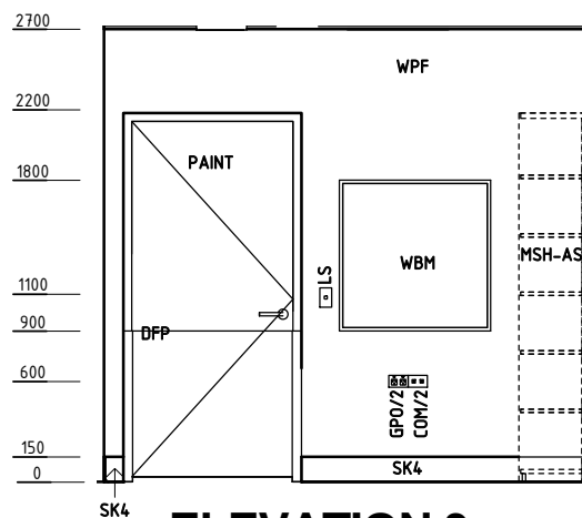
ELEVATION 3
