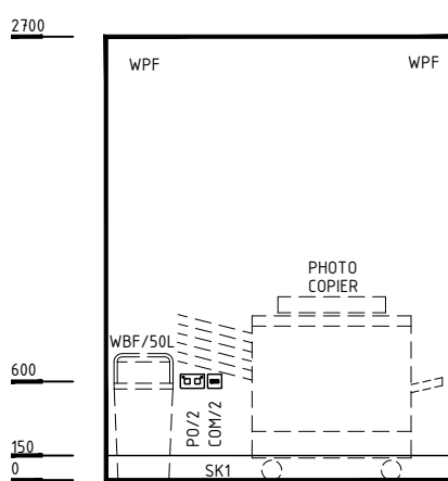
ELEVATION 3
