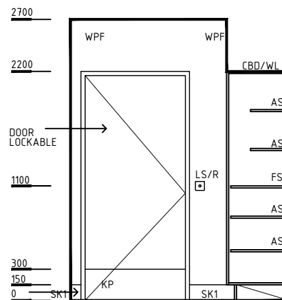
ELEVATION 4
