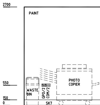
ELEVATION 1
