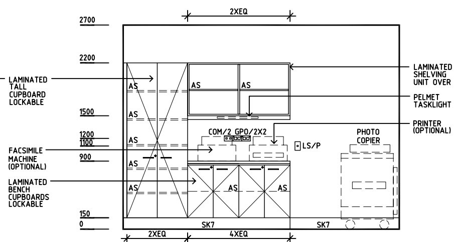
ELEVATION 4
