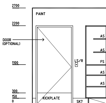
ELEVATION 3
