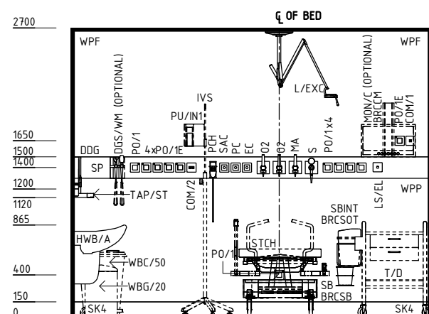
ELEVATION 4
