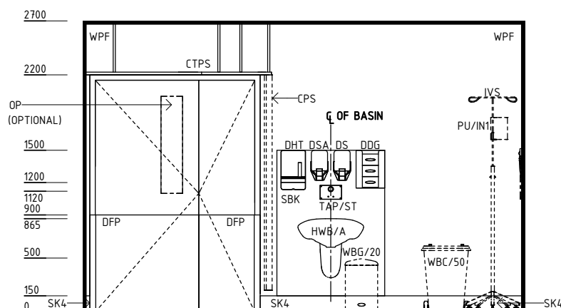
ELEVATION 3
